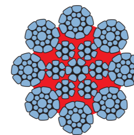
8x19 SR
