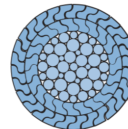
2Z 41 FWL
