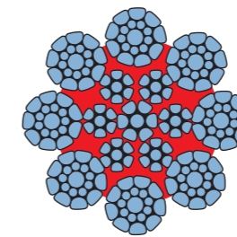
8x19 SR
