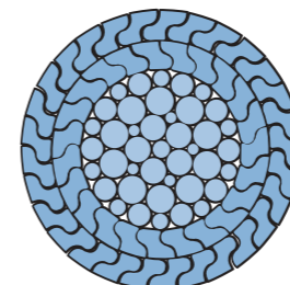
2Z 41 FWL
