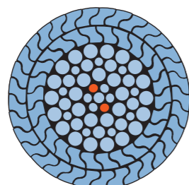
内部装有光纤维的承载索
