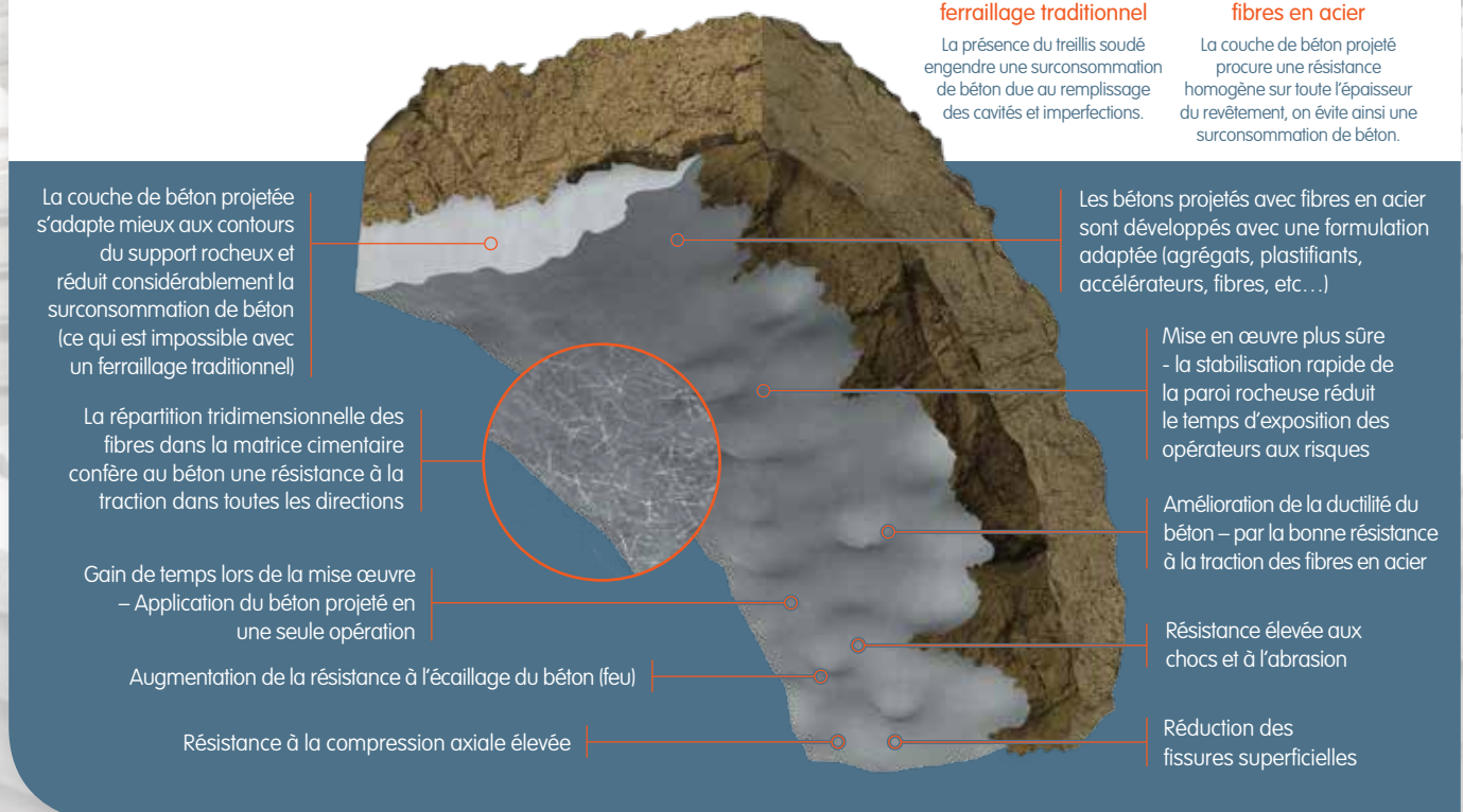
Béton projeté avec fibres en acier
